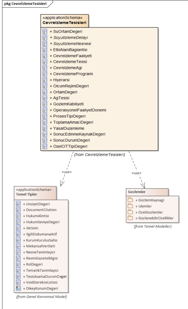
Şekil 3 UML Paket Yapısı: Çevre İzleme Tesisleri Uygulama Şemasına Genel Bakış
