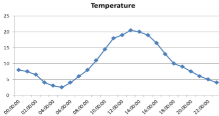
Şekil 2 Zaman Serisi Örneği
