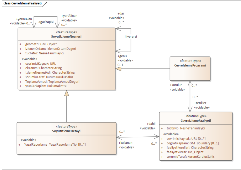
Şekil 8 UML Sınıf Diyagramı: Çevre İzleme Faaliyeti
