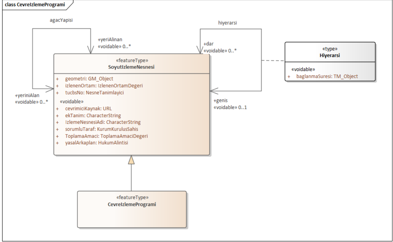
Şekil 7 UML Sınıf Diyagramı: Çevre İzleme Programı
