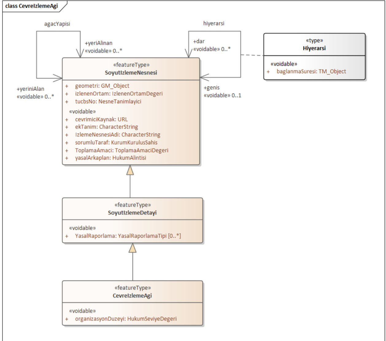
Şekil 6 UML Sınıfı Diyagramı: Çevre İzleme Ağı
