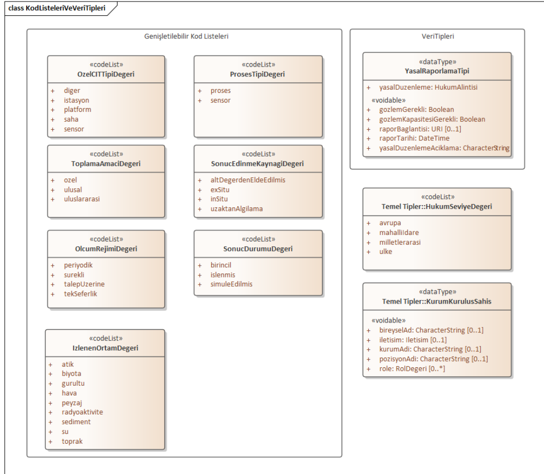
Şekil 9 UML Sınıf Diyagramı: Çevre İzleme Tesisleri Uygulama Şemasına Genel Bakış - Kod Listeleri Görünümü
