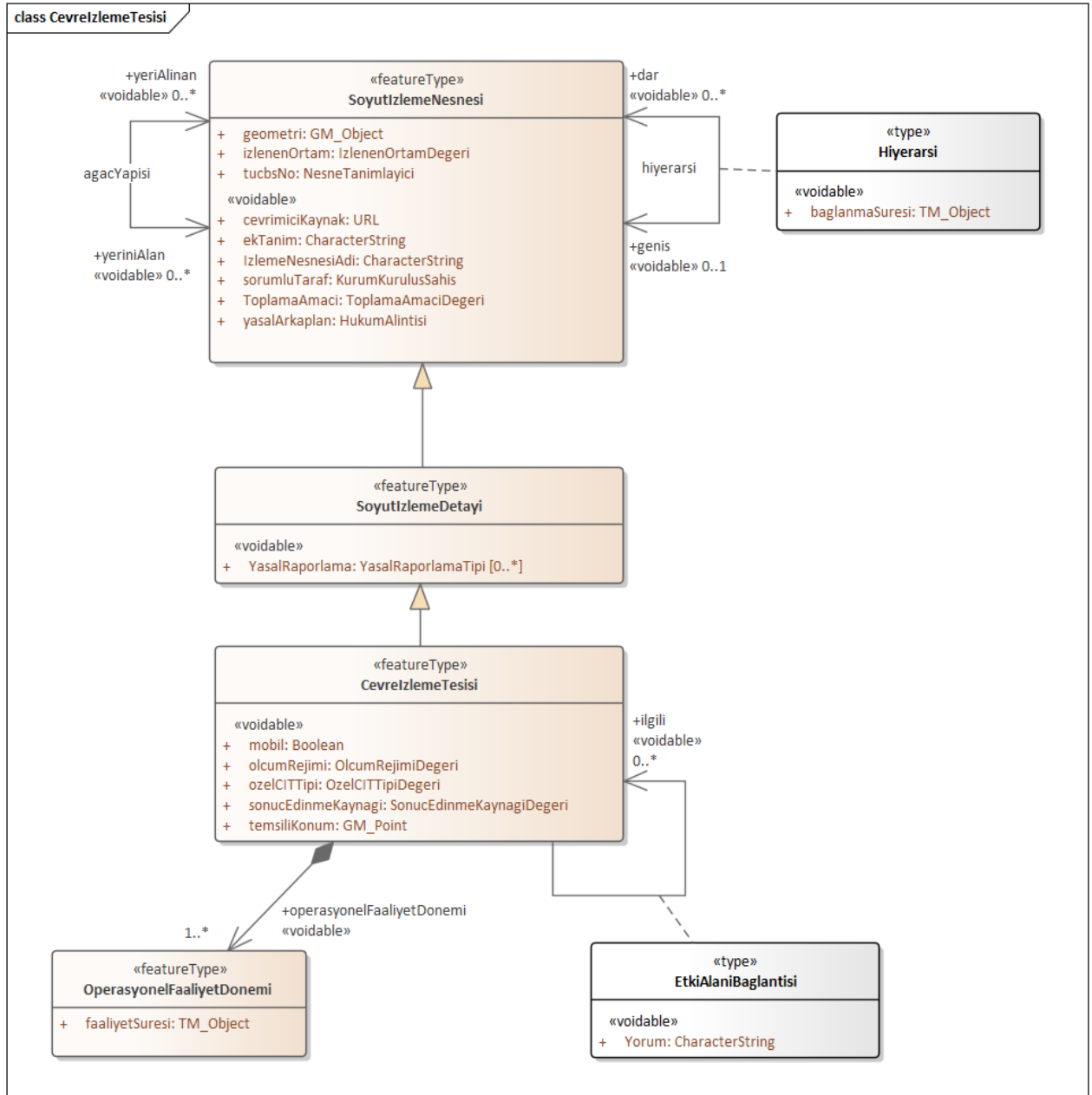
Şekil 5 UML sınıf diyagramı: Çevre İzleme Tesisleri
