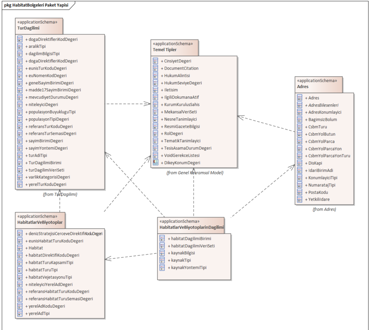
Şekil 4 UML Paket Yapısı: Habitat Bölgeleri Temasına Genel Bakış
