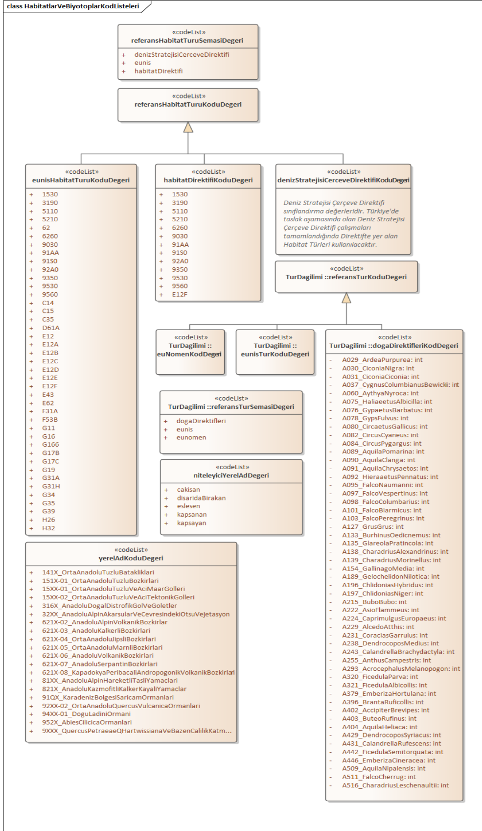
Şekil 3 UML Sınıf Diyagramı: HabitatlarVeBiyotoplar Uygulama Şeması Kod Listeleri
