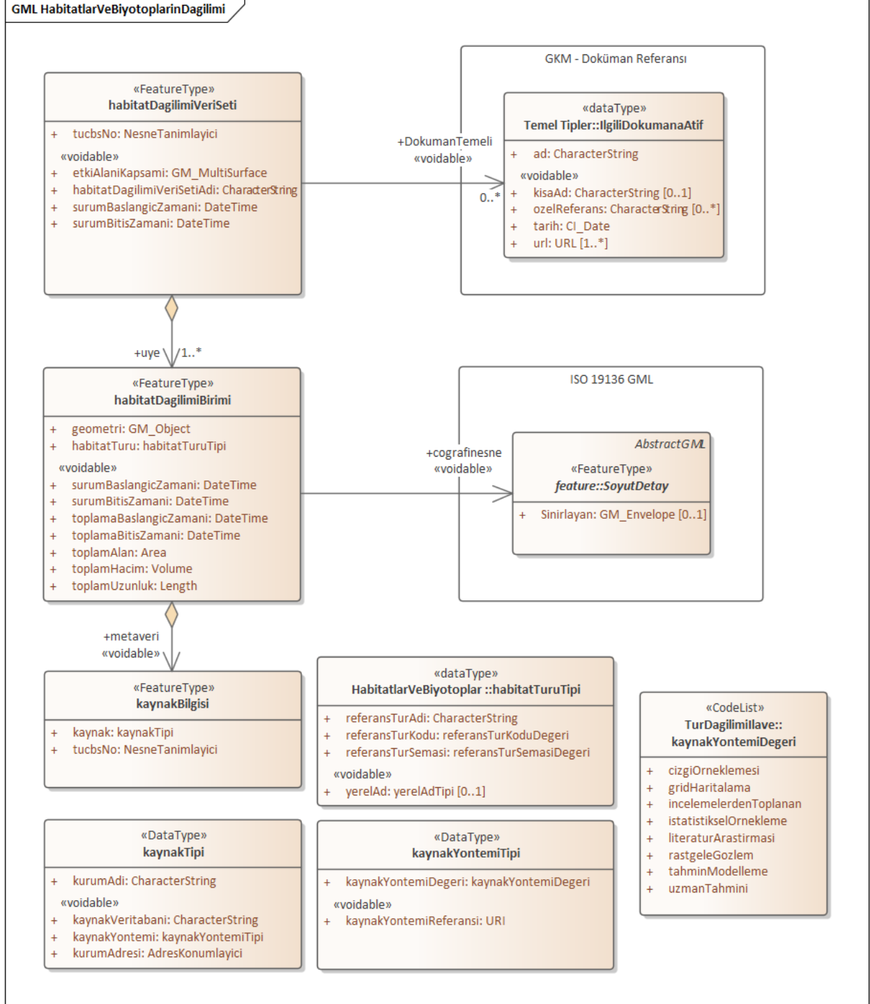
Şekil 6 UML Sınıf Diyagramı: f HabitatlarVeBiyotoplarınDagilimi Uygulama Şemasına Genel Bakış
