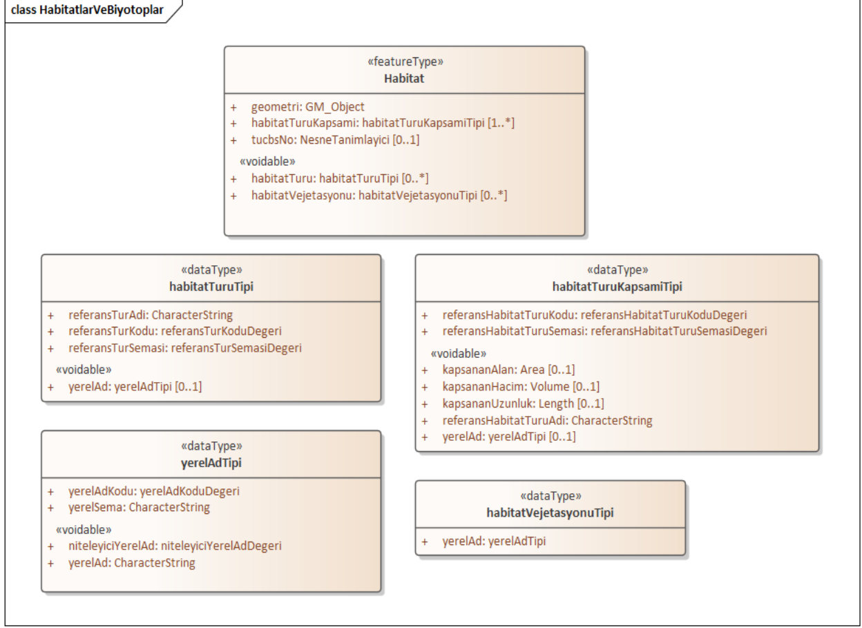
Şekil 2 UML Sınıf Diyagramı: HabitatlarVeBiyotoplar Uygulama Şeması Genel Yapısı
