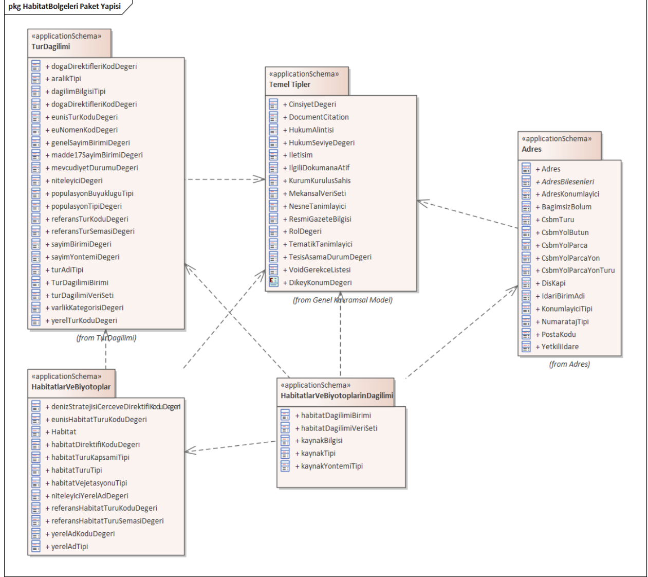
Şekil 1 UML Paket Yapısı: Habitat Bölgeleri Temasına Genel Bakış
