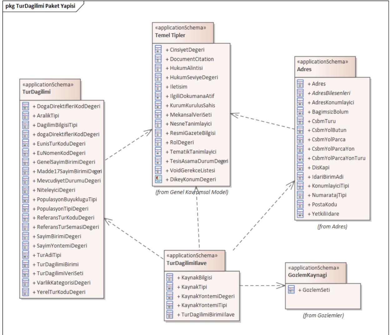
Şekil 5 UML Paket Yapısı: Tür Dağılımı Temasına Genel Bakış
