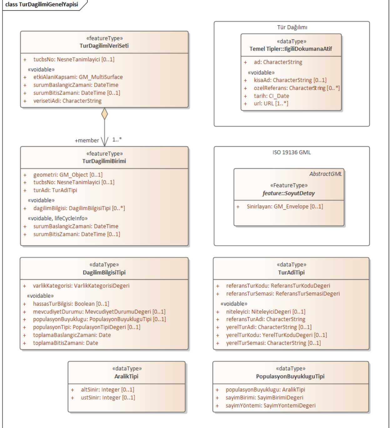
Şekil 3 UML Sınıf Diyagramı: Tür Dağılımı Uygulama Şemasına Genel Bakış
