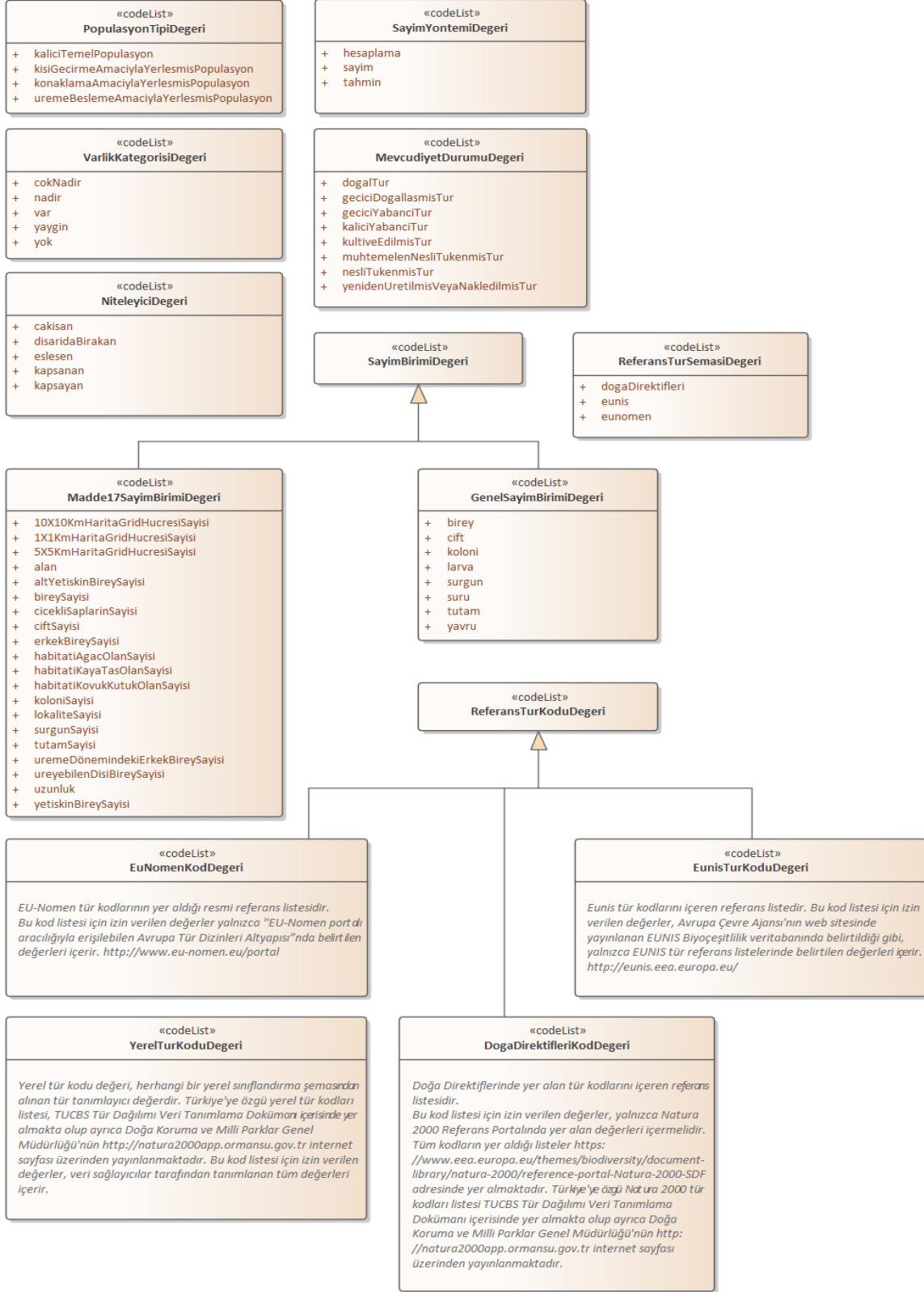
Şekil 4 UML Sınıf Diyagramı: Tür Dağılımı Uygulama Şemasına Genel Bakış (Kod Listeleri)
