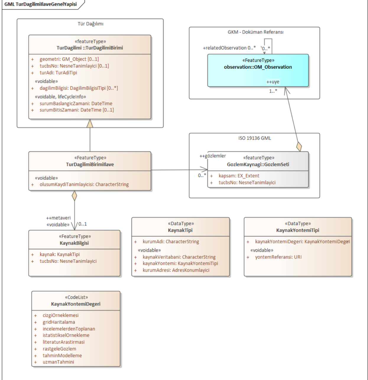
Şekil 6 UML Sınıf Diyagramı: Tür Dağılımı İlave Uygulama Şemasına Genel Bakış
