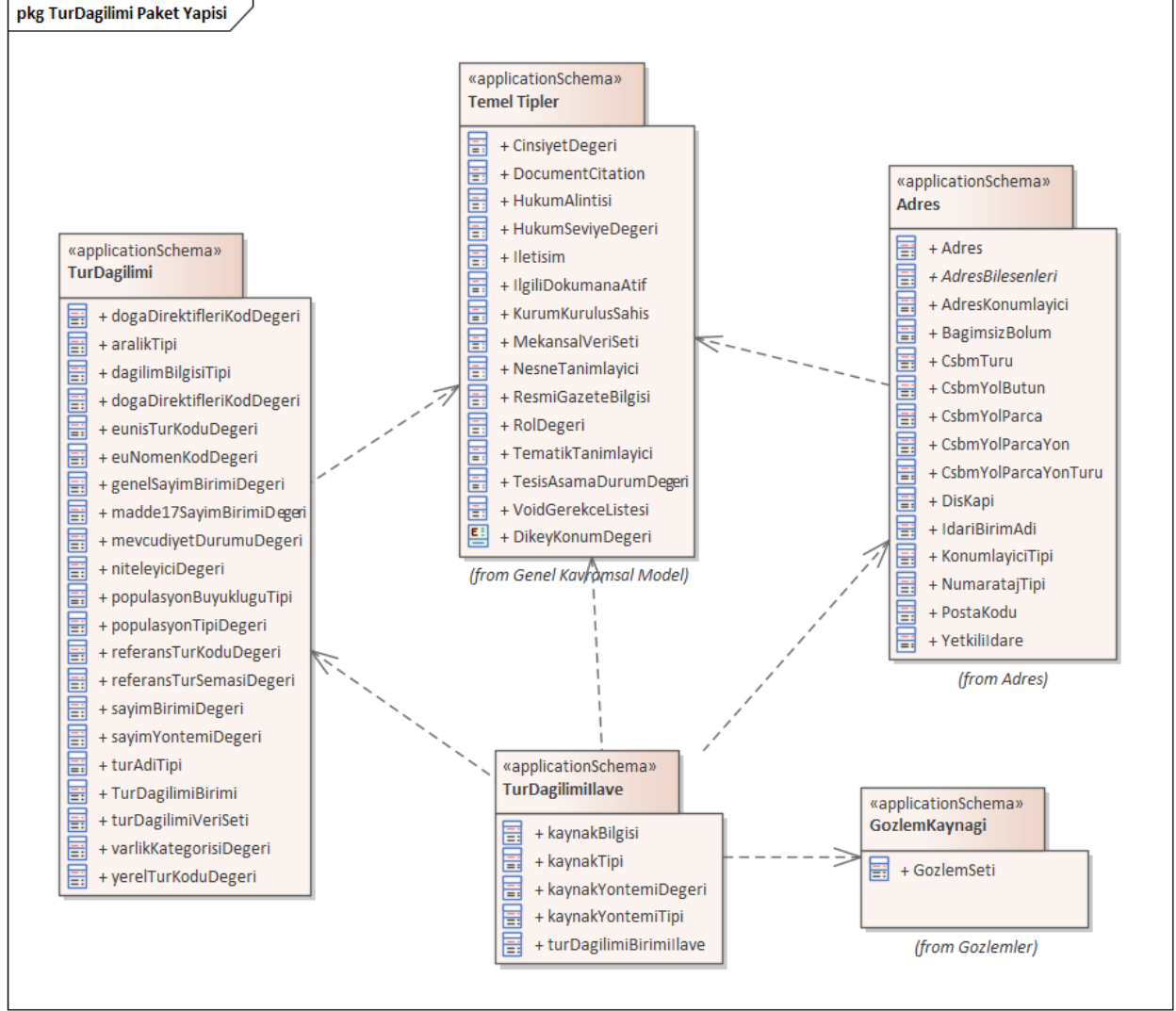
Şekil 2 UML Paket Yapısı: Tür Dağılımı Temasına Genel Bakış
